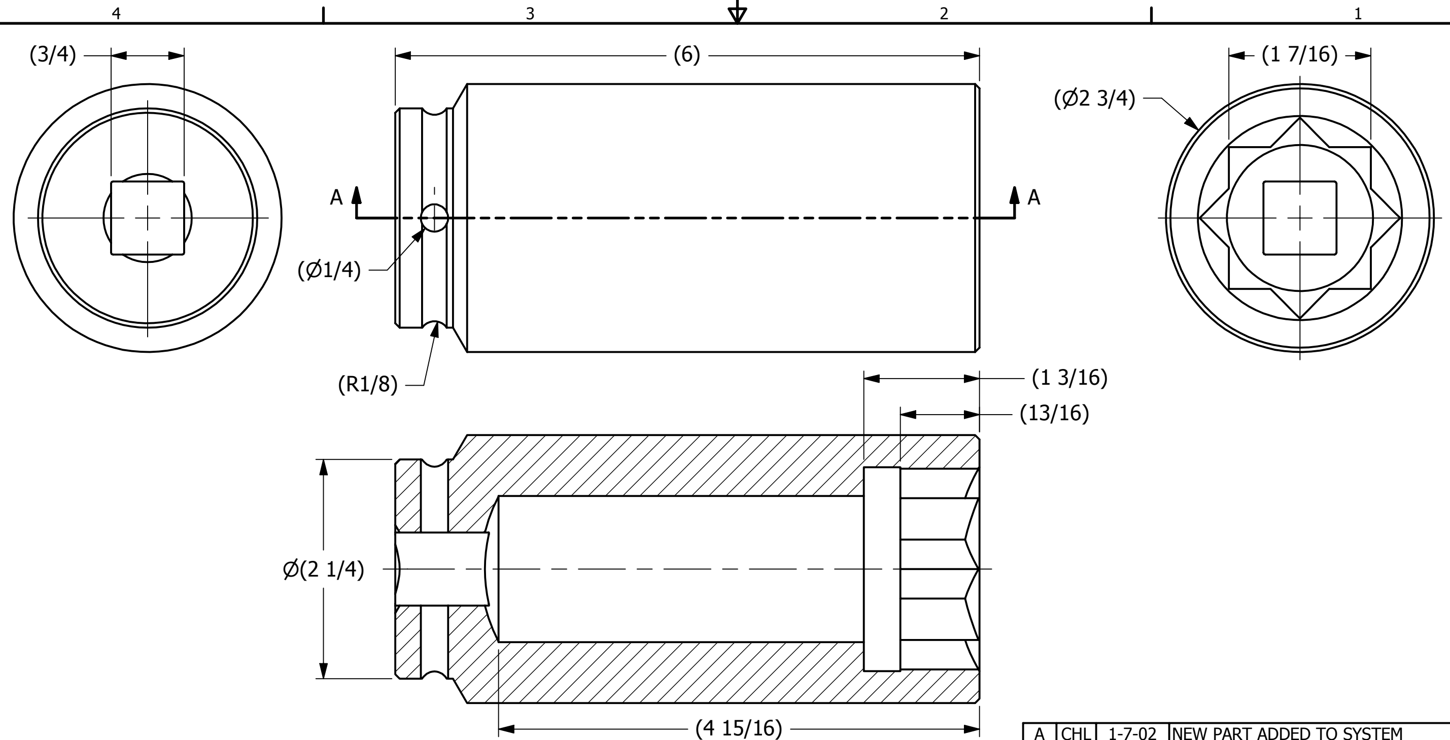
SECTION A-A
